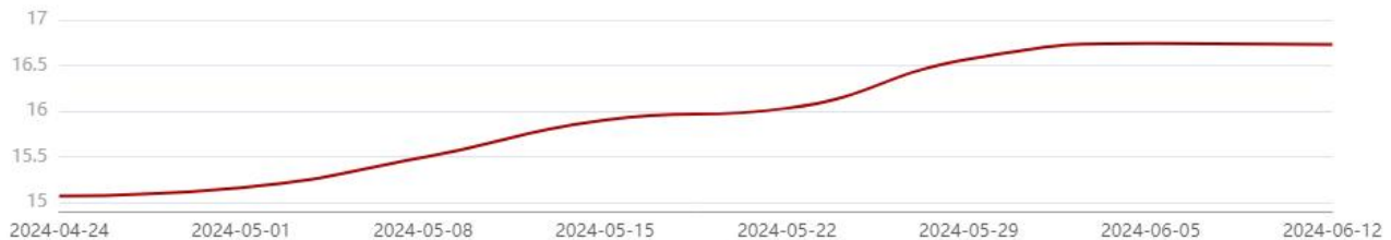
图 3、全国重点样本钢企废钢日耗量走势图
