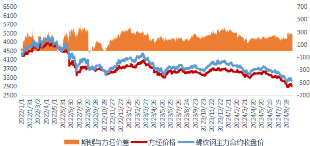
螺纹01合约与钢坯价差 (主力3078-钢坯2770=308)
