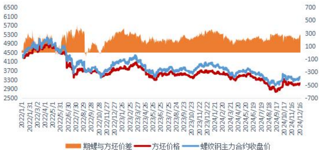
螺纹05合约与钢坯价差 (主力3364-钢坯3110=254)
